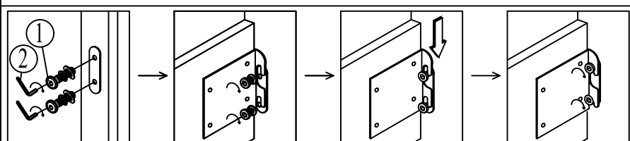
Detail-A / Détail-A
